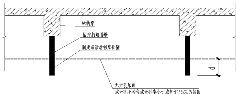
图 5.6.2-1 无开孔或 开孔不均匀或开孔率小于或等于 25% 的吊顶挡烟垂壁设置及储烟仓厚度（d）示意图
