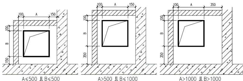
图 C-2 两面后砌墙风管安装尺寸
