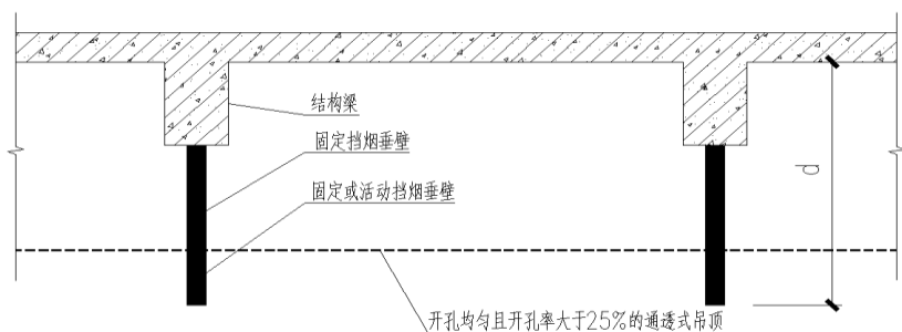
图 5.6.2-2 开孔均匀且开孔率大于 25% 的通透式吊顶挡烟垂壁设置及储烟仓厚度（d）示意图
