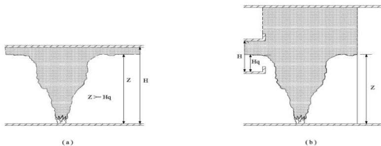
图 5.6.11-1 最小清晰高度示意图
