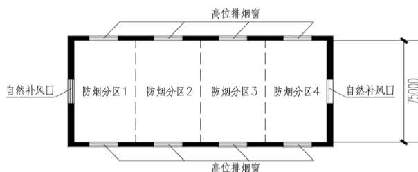
图 5.3.3 具备对流条件场所自然排烟窗的布置示意
