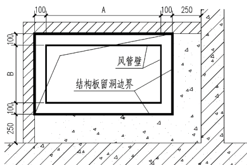
图 C-6 风井内结构楼板留洞尺寸图
